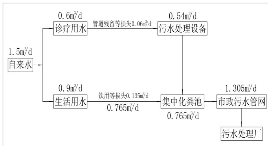
图 3 项目水平衡图
